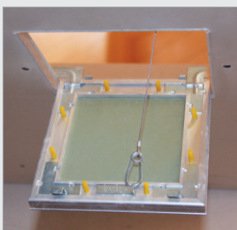
۴ نصب قاب درب دریچه
