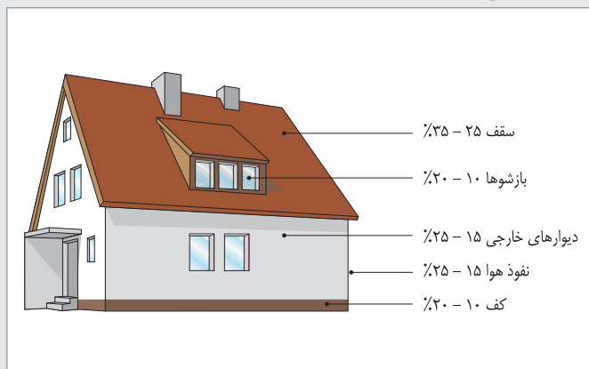
تلفات حرارتی در زمستان
