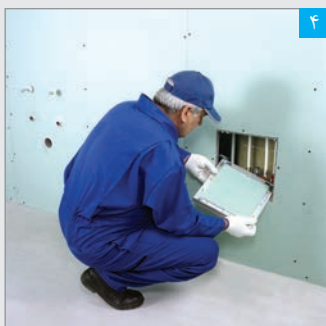
۴ نصب قاب درب دریچه
