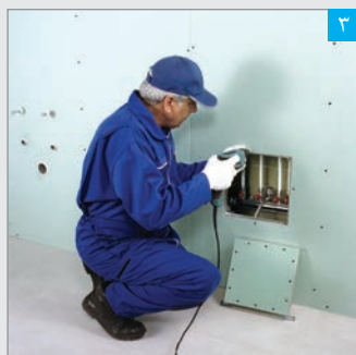
۳ قرار دادن قاب اصلی دریچه درون دیوار و پیچ کردن آن به پنل
